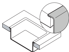
FLÄCHENBÜNDIGER EINBAU
